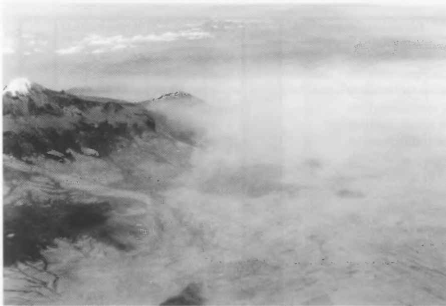
FIGURA 4.5 Contaminación en el Valle de México. El alto nivel de contaminación del aire en este valle circundado por montañas, afecta la calidad de luz en el suelo. Uno de los conos del Volcán Ixtacihuatl se ubica por arriba de la contaminación.
