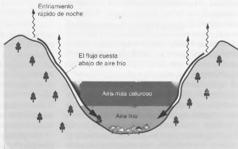
FIGURA 5.5 Descenso de aire frío y capa de inversión. El aire frío puede descender a la parte baja del valle en la noche y hacer subir una capa de aire más caliente.
